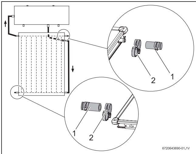
صورة 42 القامطة الشريطية الزنبركية مع حلقة الأمان والسدادة المصمتة مسبقة التركيب
