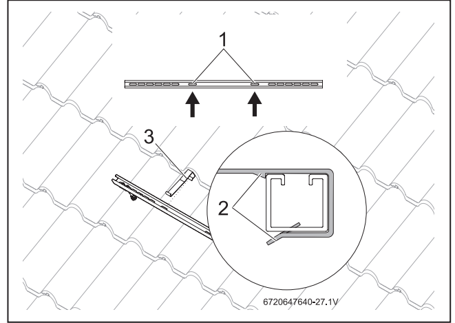
صورة 35 تعليق موانع الانزلاق
