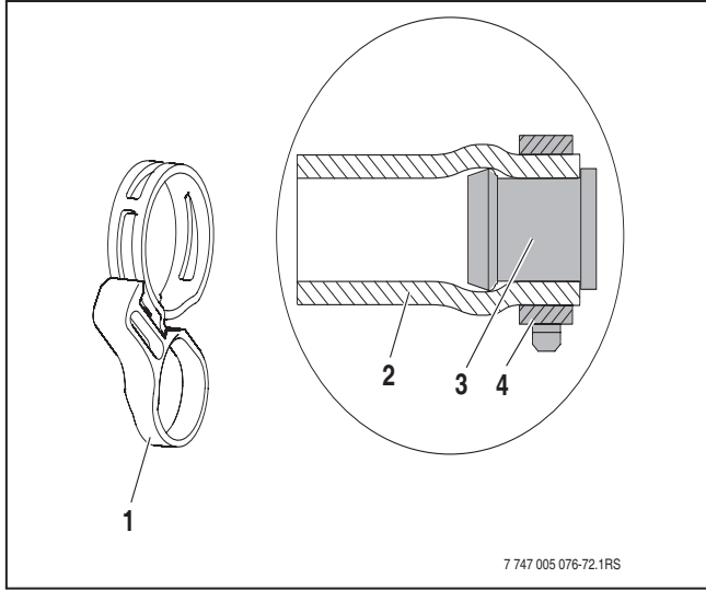
صورة 41 القامطة الشريطية الزنبركية مع حلقة الأمان والسدادة المصمتة مسبقة التركيب
