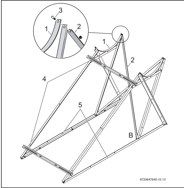
صورة 15 ربط القضبان الجانبية-U
