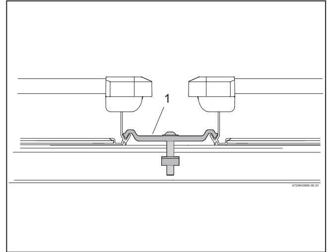
صورة 52 مشبك مجمع مزدوج بين مجموعتين
