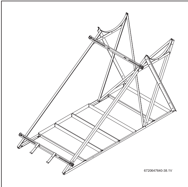
صورة 28 وصلة السقف لنظام السقف المستوي على ألواح خرسانية، القياسات بالمللي متر (هنا مع نظام 150/200-1)
